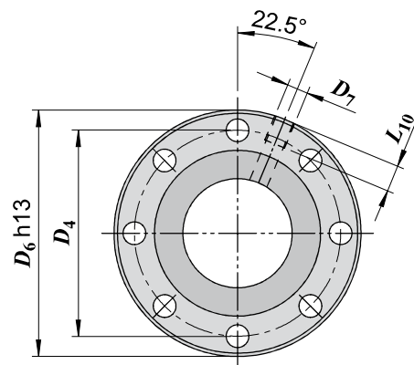
Фланец тип 2
