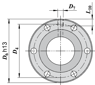
Фланец тип 1
